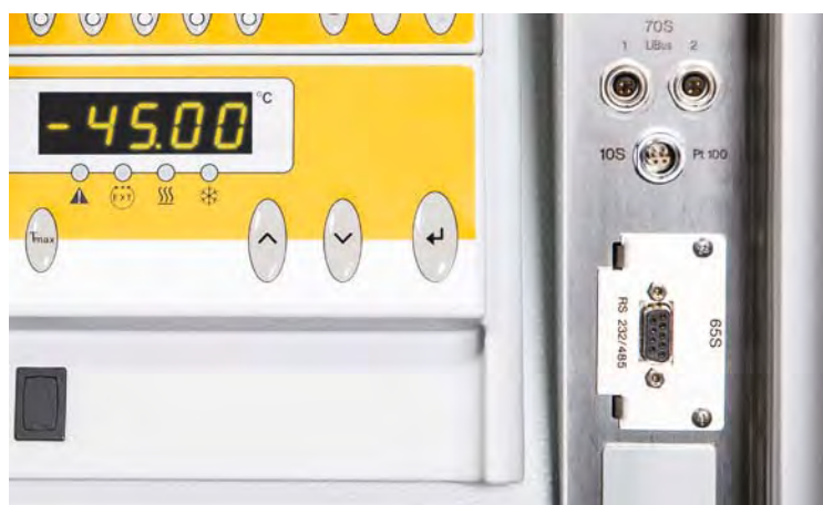
Interface RS 232/485 en série et deux autres emplacements destinés à des modules d'interfaces pour une intégration flexible dans un système
